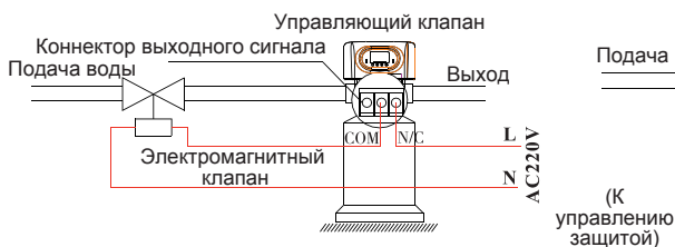
Рис. 3-2 Цепь управления электромагнитным клапаном на входе
